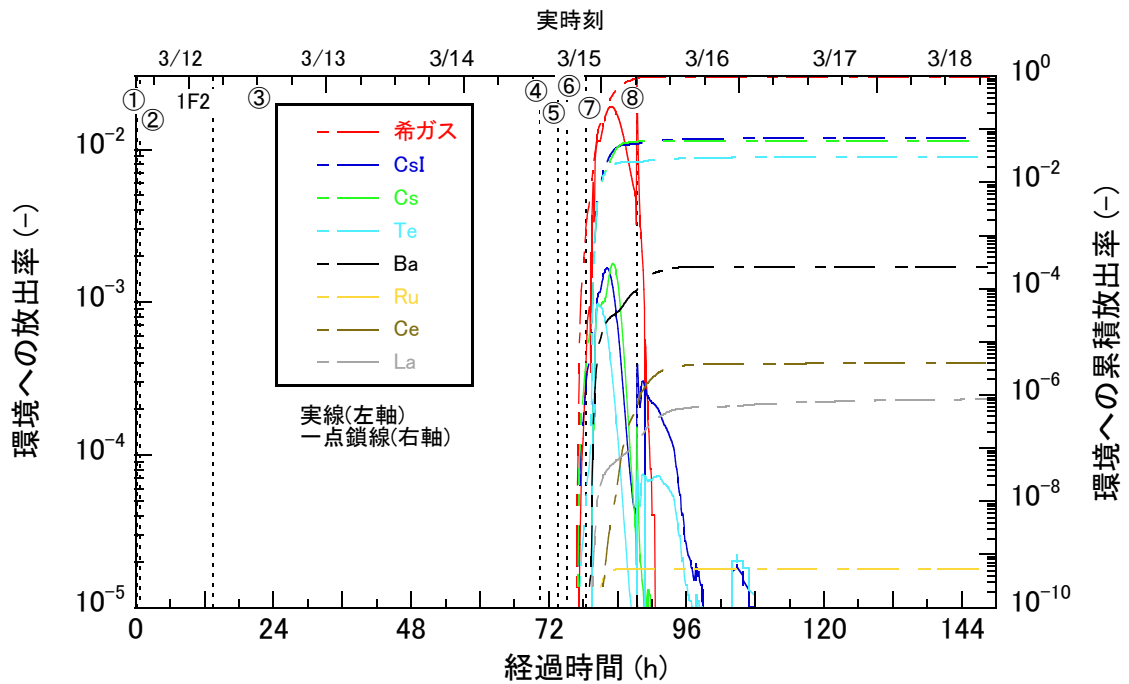
図 2-2-10 事業者解析 2 での FP 放出割合(2/2)(2号機)
